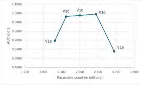
(a) AUC vs Parameter Count
