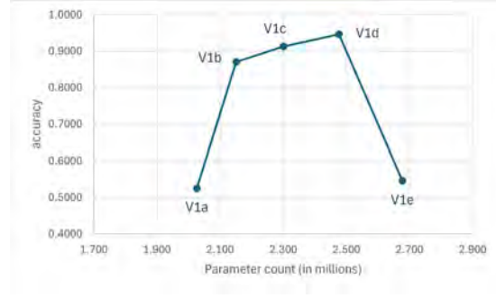
(b) Accuracy vs Parameter Count
