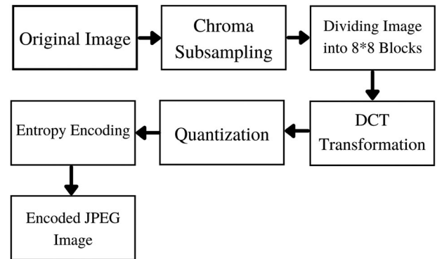
Fig. 1. JPEG encoding technique.
