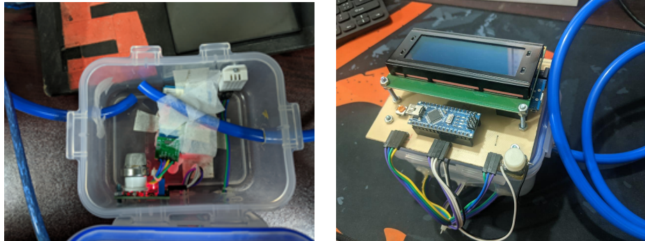
Figure19:Data collection box ( PMS7003,DHT22,MQ131)
